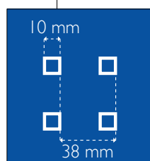
Perforations carrées 10 x 10 mm au pas de 38 mm
